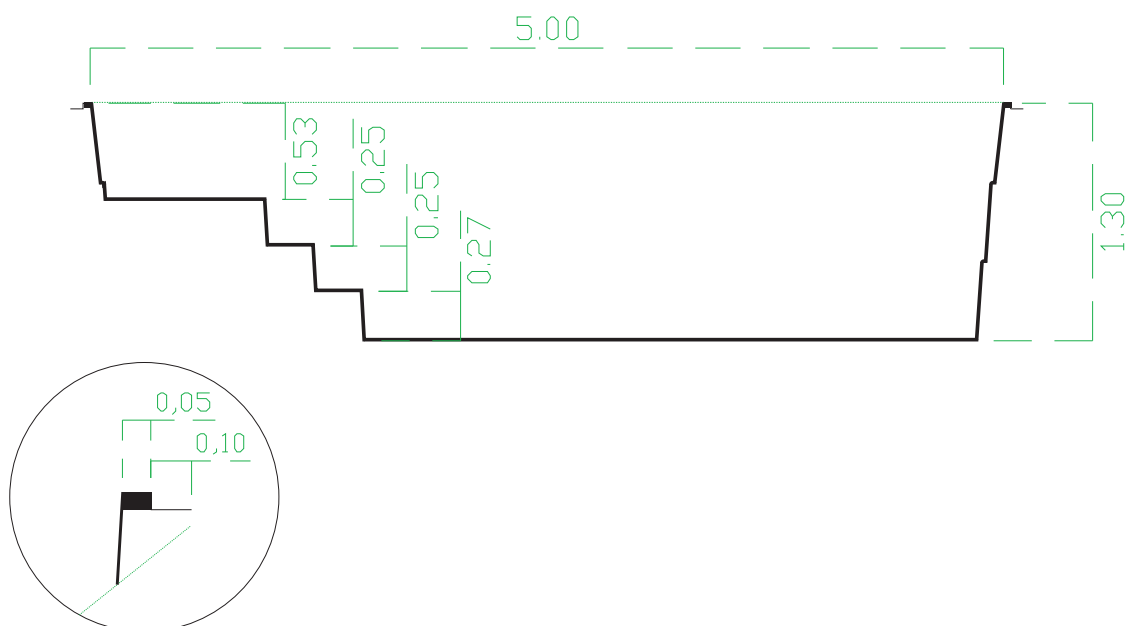
Detalhe da borda rebaixada
